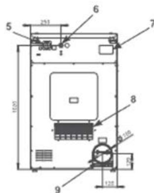
Πίσω όψη
